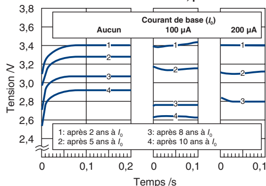
Écoulement tension à +25 °C, pulse: 120 mA
