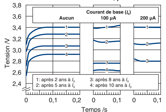
Écoulement tension à +25 °C, pulse: 120 mA
